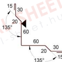
ST 018 - Merevített belső sarokszegély T=250mm
