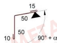
ST 068 - Tompaszögű belső sarokszegély \alpha = Tetőhajlás szöge, T=125mm
