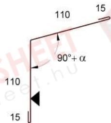
ST 006 - Tompaszögű sarokszegély \alpha = Tetőhajlás szöge, T=250mm
