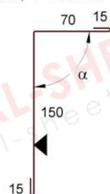
ST 026 - Eltérő szárú belső sarokszegély
