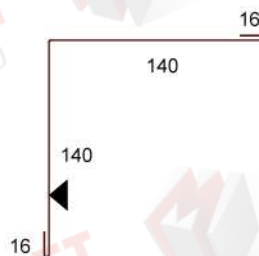
ST 008 - Derékszögű sarokszegély T=312mm
