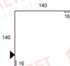
ST 007 - Derékszögű sarokszegély T= 312mm
