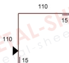
ST 001 - Derékszögű sarokszegély T= 250mm
