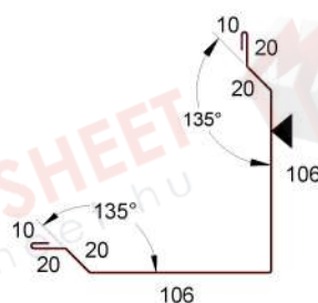
ST 014 - Merevített külső sarokszegély T=312mm
