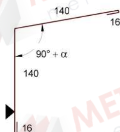
ST 011 - Tompaszögű sarokszegély \alpha = Tetőhajlás szöge, T=312mm
