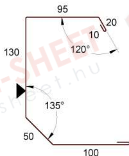
ST 045 - Oromszegély 120mm-es tetőpanelhez T= 416mm
