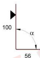
ST 024 - Merevítetlen külső sarokszegély \alpha < 180^\circ , T= 156mm
