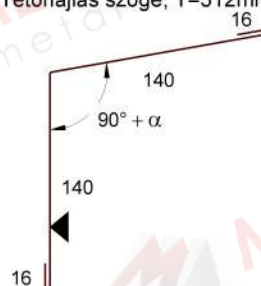
ST 012 - Tompaszögű sarokszegély \alpha = Tetőhajlás szöge, T=312mm
