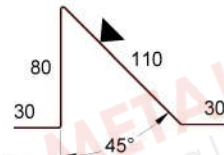
ST 078 - Hófogó szegély T=250mm
