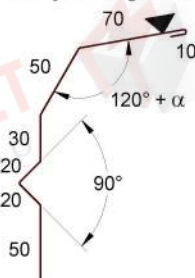
ST 061 - Ereszvég takarószegély \alpha < 30^\circ Tetőhajlás szöge, T=250mm
