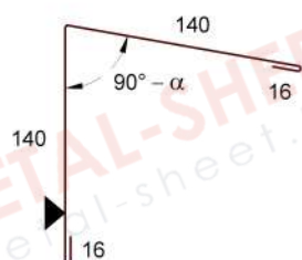
ST 009 - Hegyesszögű sarokszegély \alpha = Tetőhajlás szöge, T=312mm
