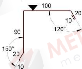
ST 058 - Oromszegély T=250mm
