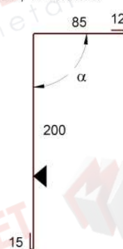
ST 028 - Eltérő szárú belső sarokszegély
