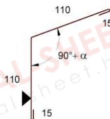
ST 005 - Tompaszögű sarokszegély \alpha = Tetőhajlás szöge, T=250mm
