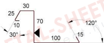
ST 057 - Oromszegély T= 250mm
