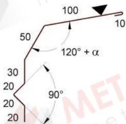
ST 060 - Ereszvég takarószegély \alpha < 30^\circ Tetőhajlás szöge, T= 250mm
