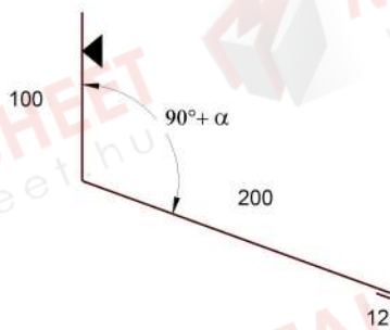
ST 022 - Fali takarószegély \alpha = Tetőhajlás szöge, T=312mm
