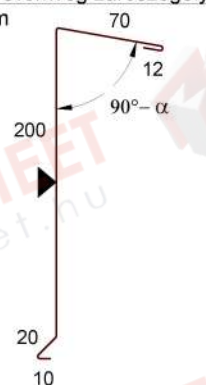
ST 046 - Oromvég zárószegély T=312mm
