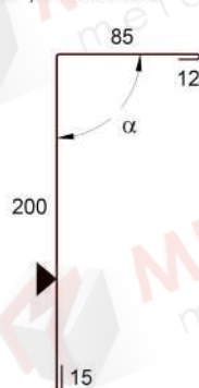
ST 027 - Eltérő szárú külső sarokszegély
