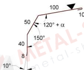
ST 062 - Ereszvég takarószegély \alpha < 30^\circ Tetőhajlás szöge, T=250mm
